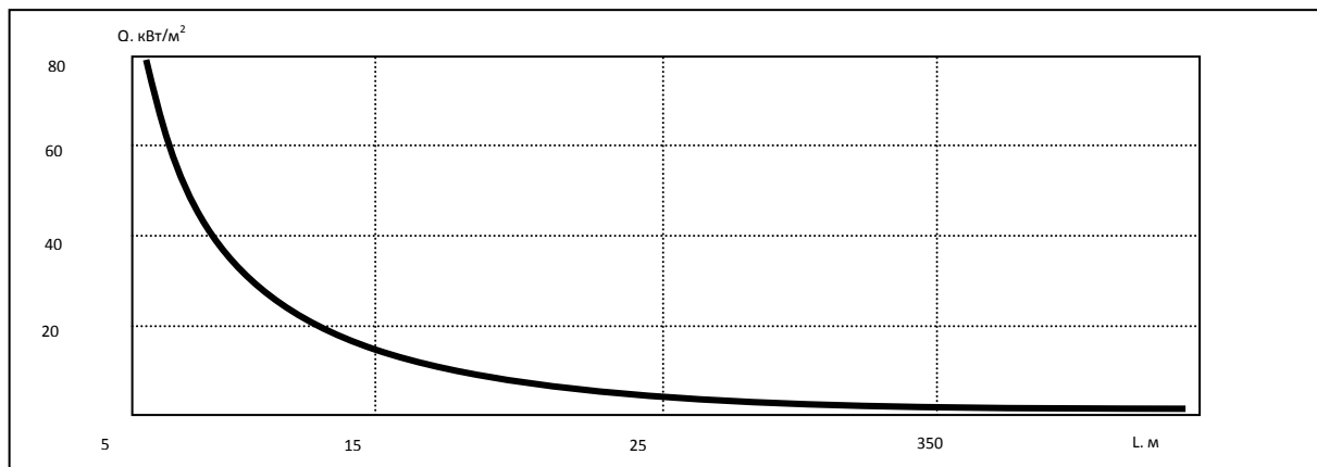
Рис. 3.2.4. Зависимость плотности теплового потока C при горении зданий I-III степени огнестойкости
